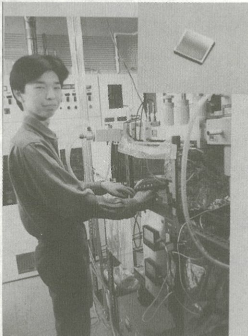
■ダイヤモンド薄膜成長(木村・斎藤・湯郷研究室) プラズマCVDというこの装置は電子レンジの大きなもの、いわば「ダイヤモンドの調理器具」です。これによって、新しい半導体素子としての応用が期待されるダイヤモンドの薄膜(右上)が出来上がります。
