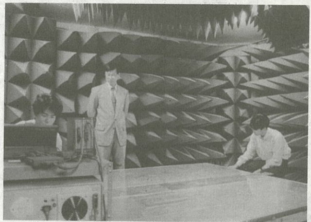
■電波暗室でのアンテナの特性測定(岩崎・石上研究室) この奇妙な部屋はいわば「電波の無響室」で、アンテナの特性測定には欠かせません。ここでは妨害電波を測定するためのアンテナの特性を測っています。
