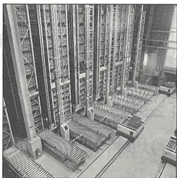
AS/RS高速小型立体自動倉庫 〈ファインストッカー〉
